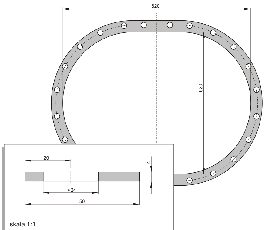
rys.1 skala 1:10
